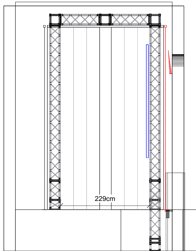
Schnitt 1 - Seitenansicht
